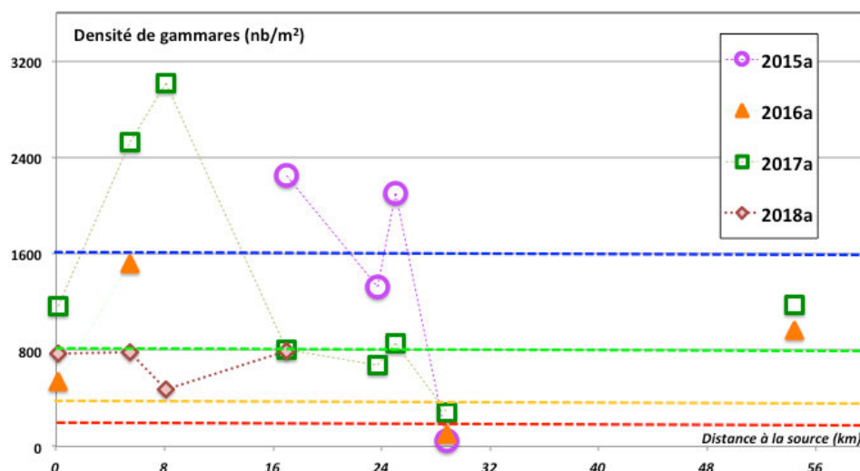
Figure 8. Variations spatio-temporelles de l'abondance de gammarès mesurées en fin de période estivale, en septembre ou en octobre, sur les stations jalonnant la Loue. Les lignes en pointillé signalent les seuils de densités très faible (rouge), faible (jaune), moyen (vert) et fort (bleu), établis à partir des moyennes de densités observées sur plusieurs centaines de stations prospectées à l'aide du même protocole (MAG20)
