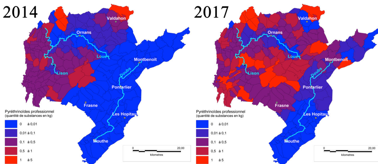
Figure 24. Evolution de la quantité de pyréthrinoïdes achetés et potentiellement utilisés dans les différents cantons composant le bassin versant Haut-Doubs Haute-Loue (périmètre du SAGE)
