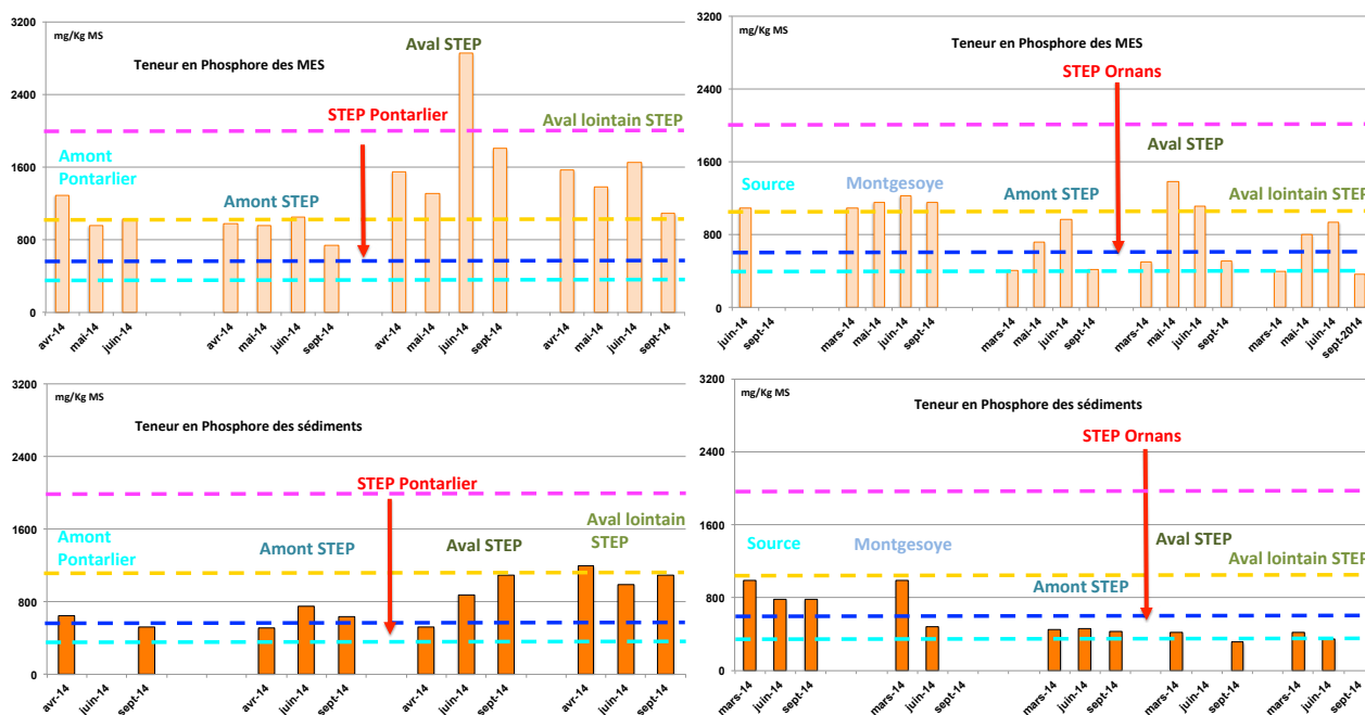
Figure 13. Comparaison des teneurs en phosphore des sédiments et des matières en suspension prélevées à plusieurs occasions dans le Doubs à l'amont et à l'aval de l'agglomération Pontisallienne (à gauche) et dans la source de la Loue ainsi qu'à l'amont et à l'aval de l'agglomération d'Ornans (à droite)
