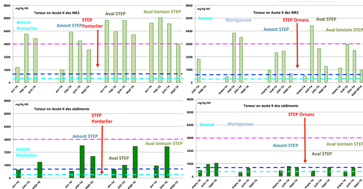
Figure 14. Comparaison des teneurs en azote des sédiments et des matières en suspension prélevées à plusieurs occasions dans le Doubs à l'amont et à l'aval de l'agglomération de Pontarlier (à gauche) et dans la source de la Loue ainsi qu'à l'amont et à l'aval de l'agglomération d'Ornans (à droite)
